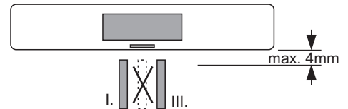
Der runde Stabmagnet kann auch ohne Magnetgehäuse montiert werden. Damit besteht die Möglichkeit den Magneten direkt in Bohrungen von Holzfenstern zu integrieren. Bitte beachten Sie dabei, dass der Magnet seitlich der Reedkontakt Markierung montiert ist! (Position I. oder III. - Position II. ist nicht zulässig)
